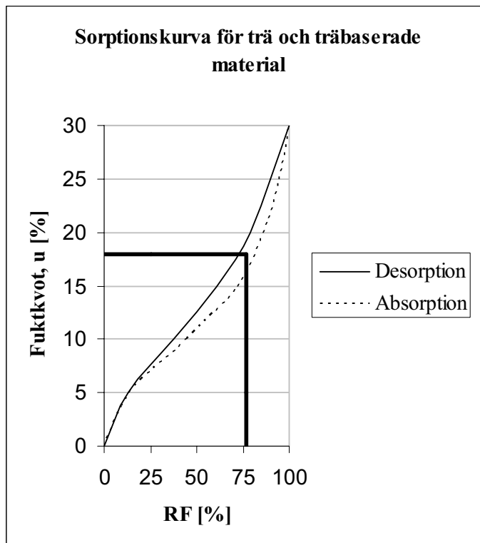
Figur 3.4 Diagrammet visar en generell sorptionskurva för trämaterial där relationen mellan materialets fuktkvot och luftens relativa fuktighet kan utläsas. Egen bearbetning (Pettersson, 2004).
